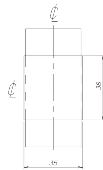
패널커버 절단 치수
