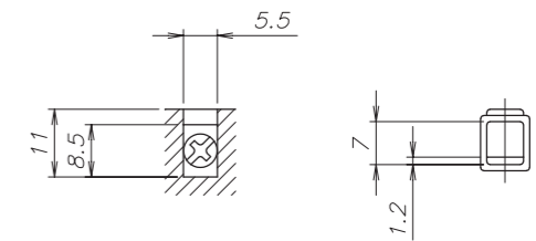
■ 단자부 상세도
